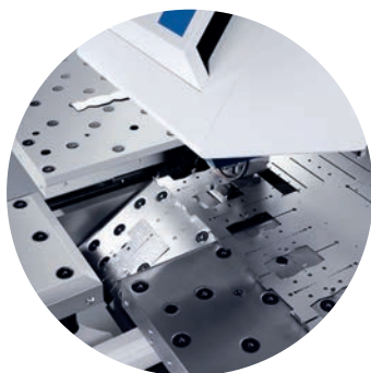
Изготовление деталей на координатно-пробивном прессе с ЧПУ
